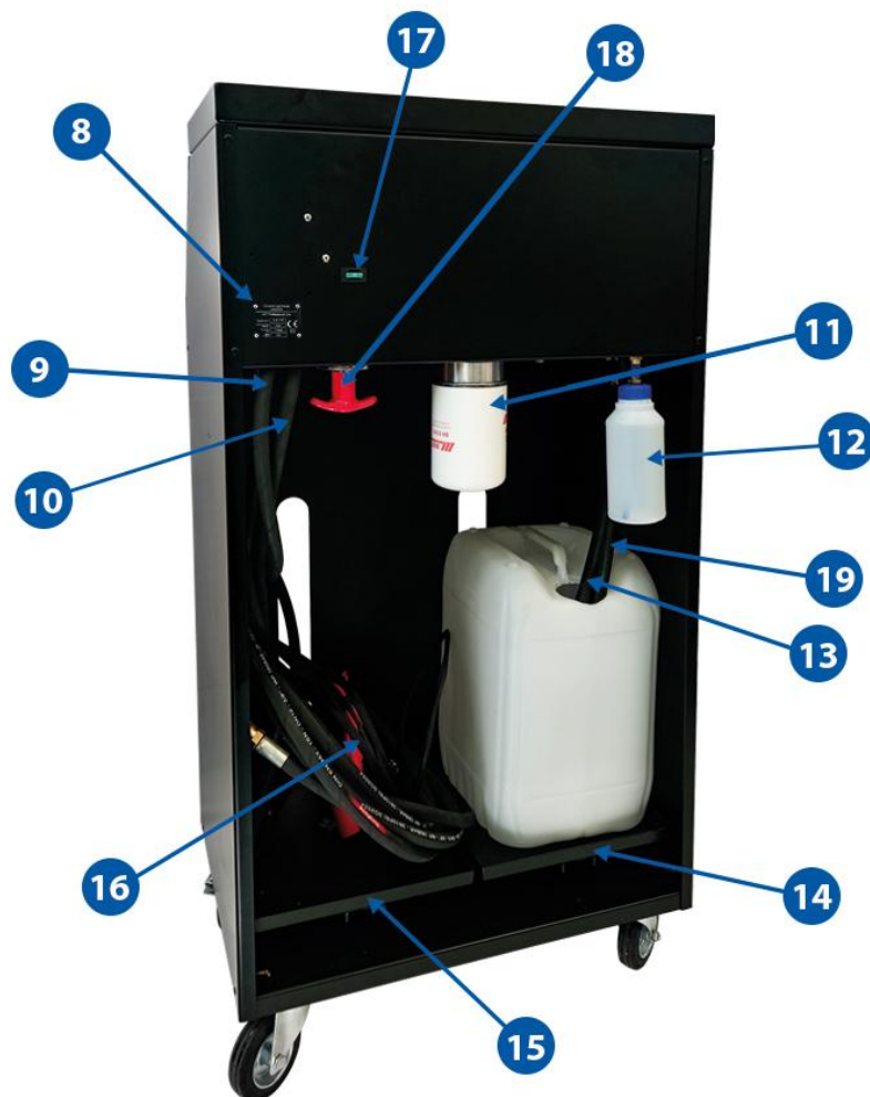
Figura 2. Vista trasera del equipo
